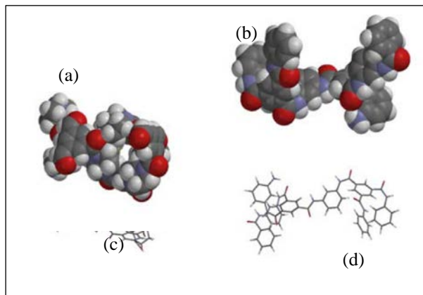
Rajah 14 Model pengisian ruang: (a) PIP-TMC poliamida, (b) BA-TMC poliamida, dan tiub model bagi (c) PIP-TMC poliamida dan (d) BA-TMC poliamida
